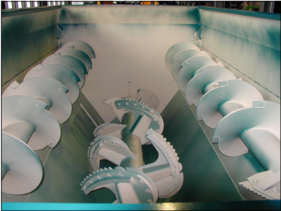
Agitateur médian et vis de recyclage latérales
